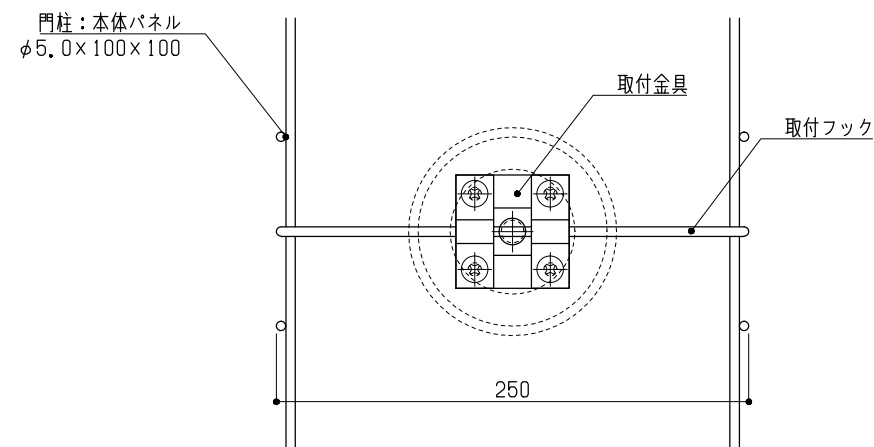
平面図 S = 1 : 4
