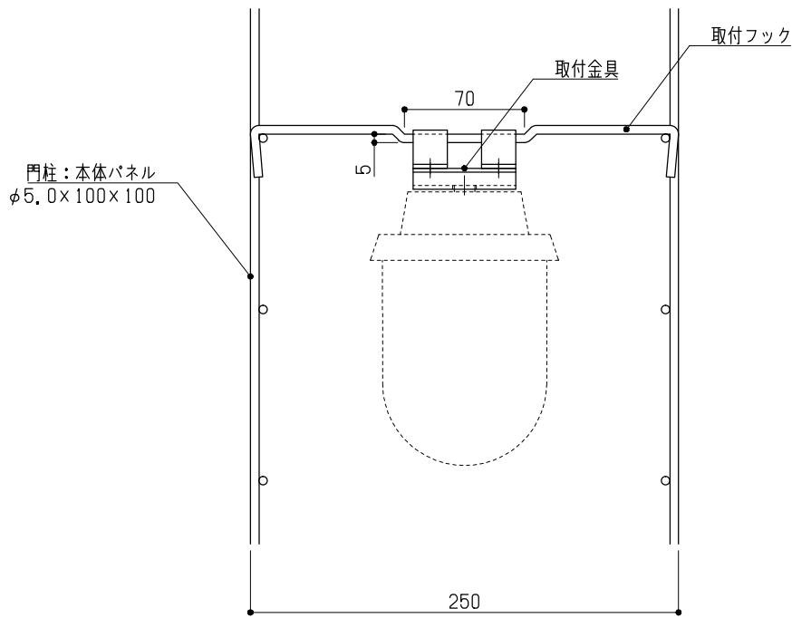
正面図 S = 1 : 4
