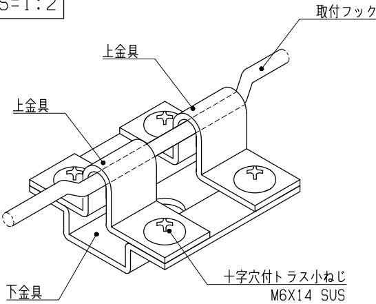
金具組立図 S=1：2
