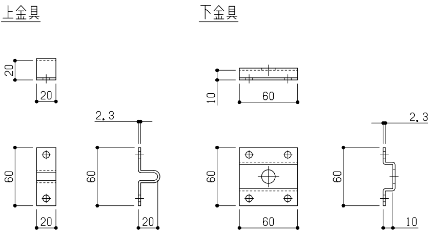
照明取付金具 詳細図 S=1：4
